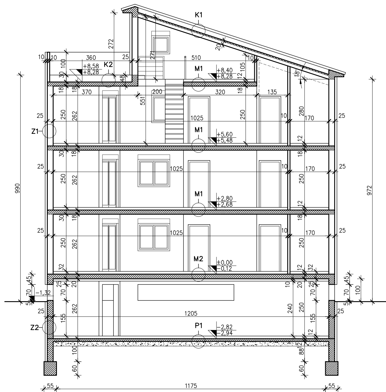
PRESJEK 1-1
