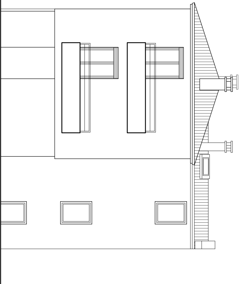
ZAPADNO PROČELJE
