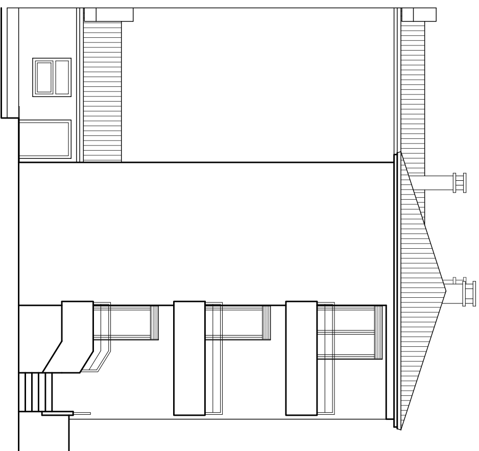
ISTOČNO PROČELJE
