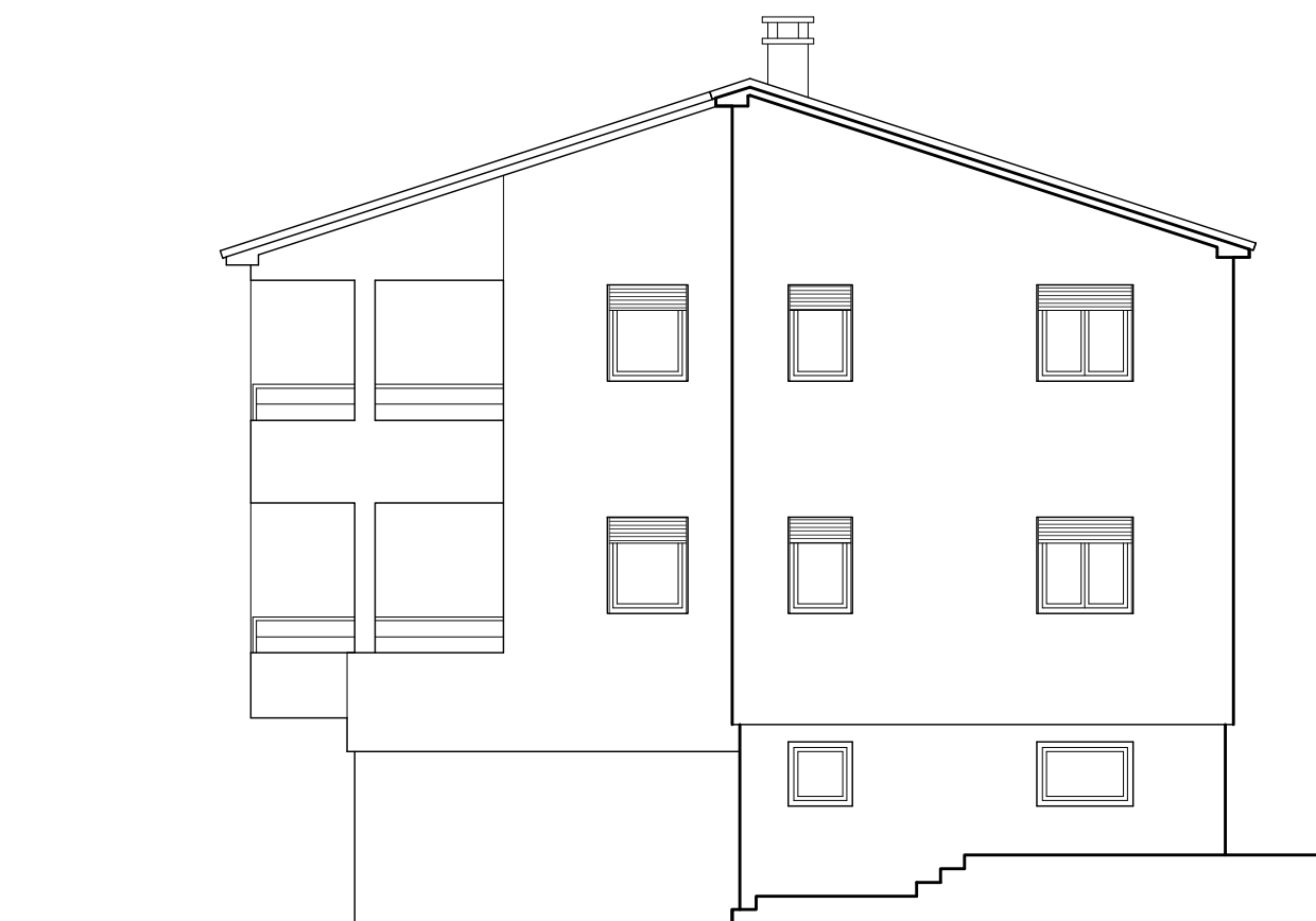
ISTOČNO PROČELJE
