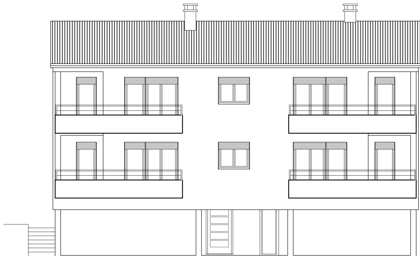
JUŽNO PROČELJE
