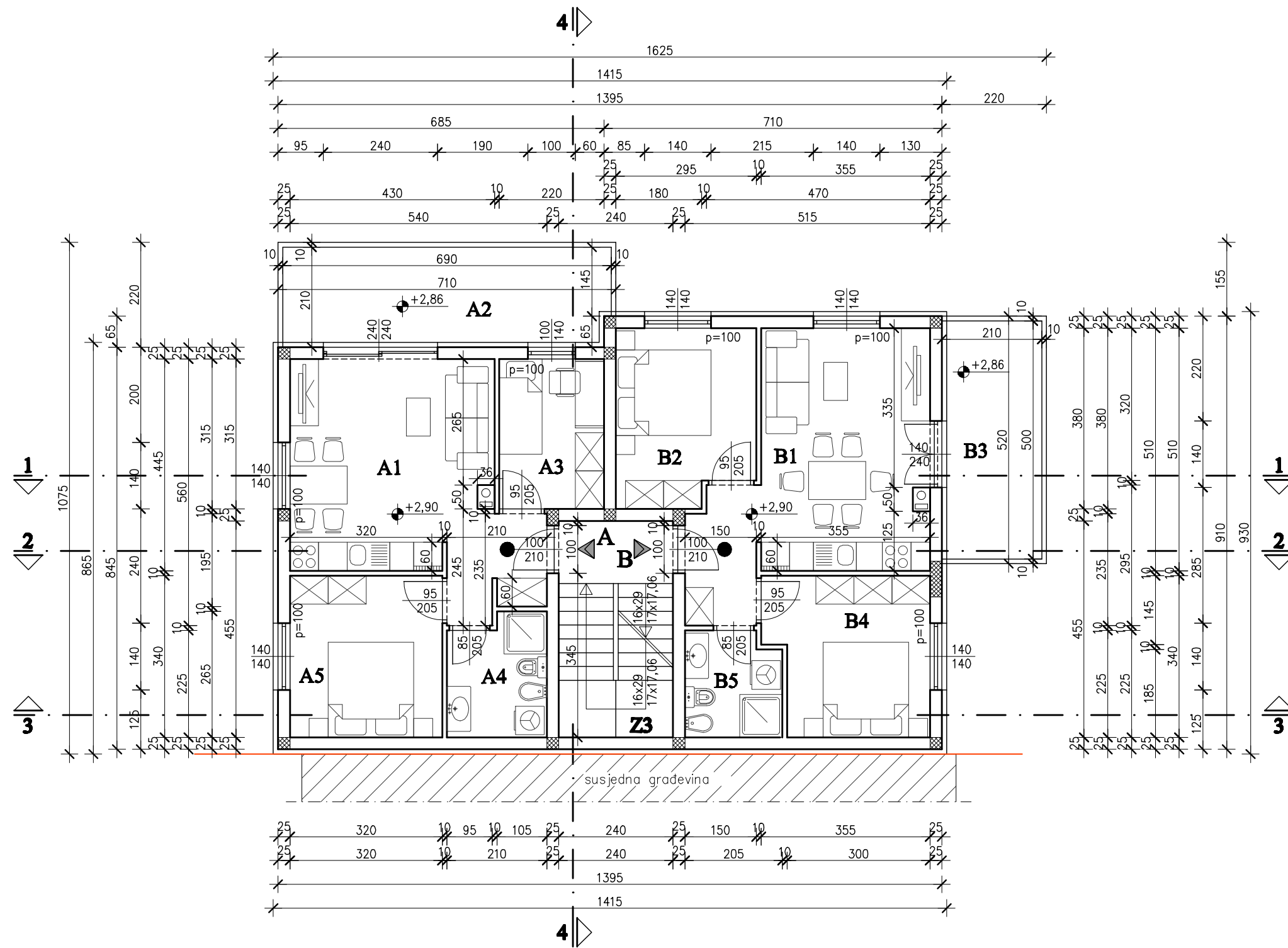
ISKAZ NETO POVRŠINA PRVOG KATA
