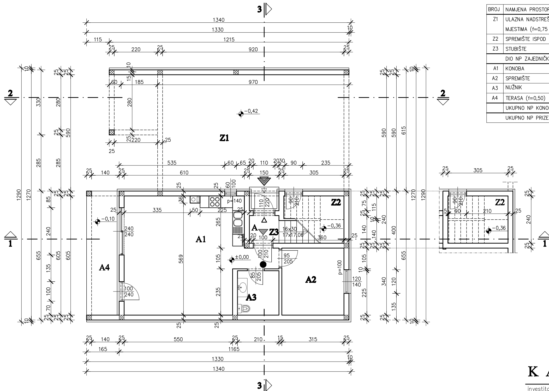
ISKAZ NETO POVRŠINA PRIZEMLJA
