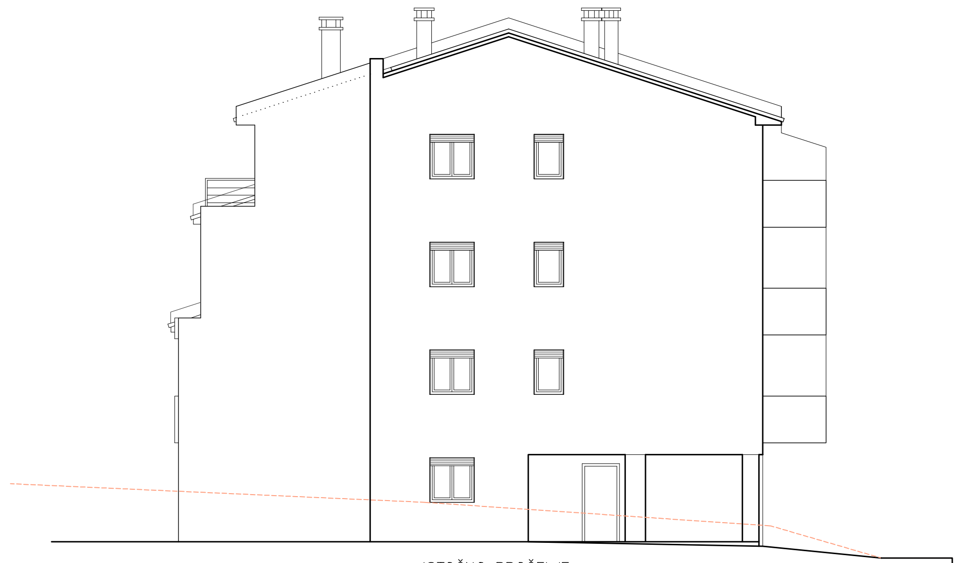
ISTOČNO PROČELJE
