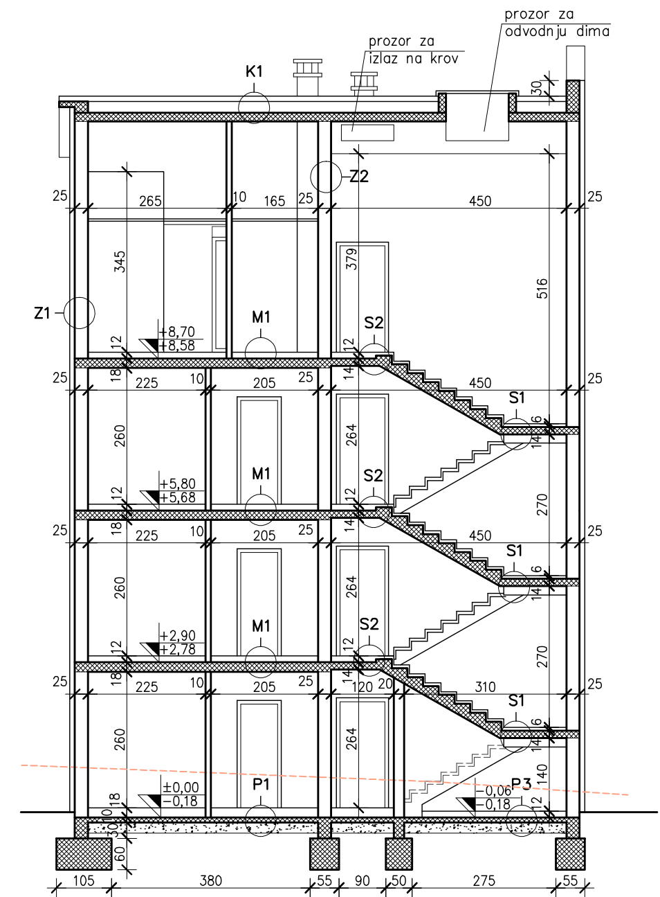
PRESJEK 4-4
