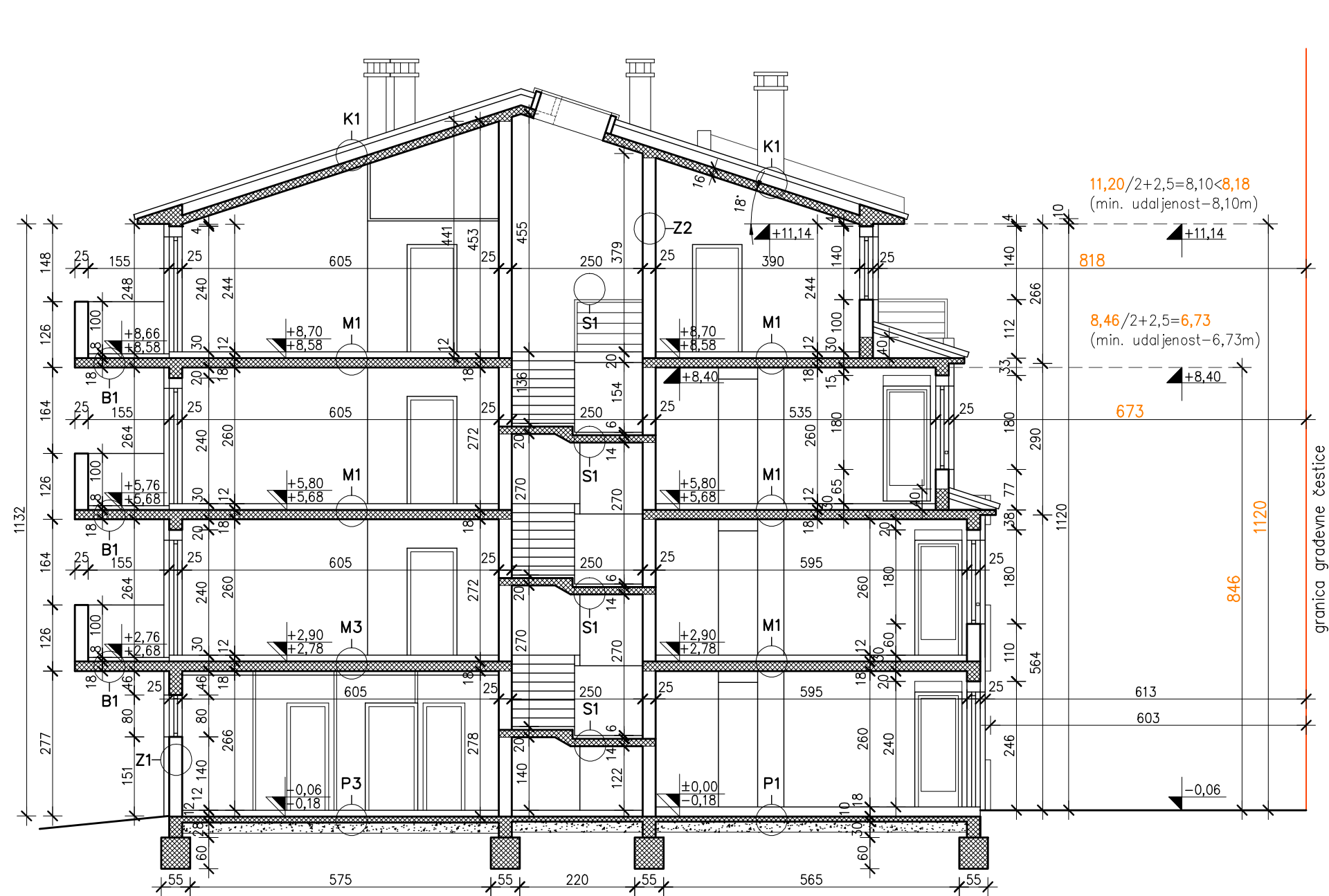
PRESJEK 3-3
